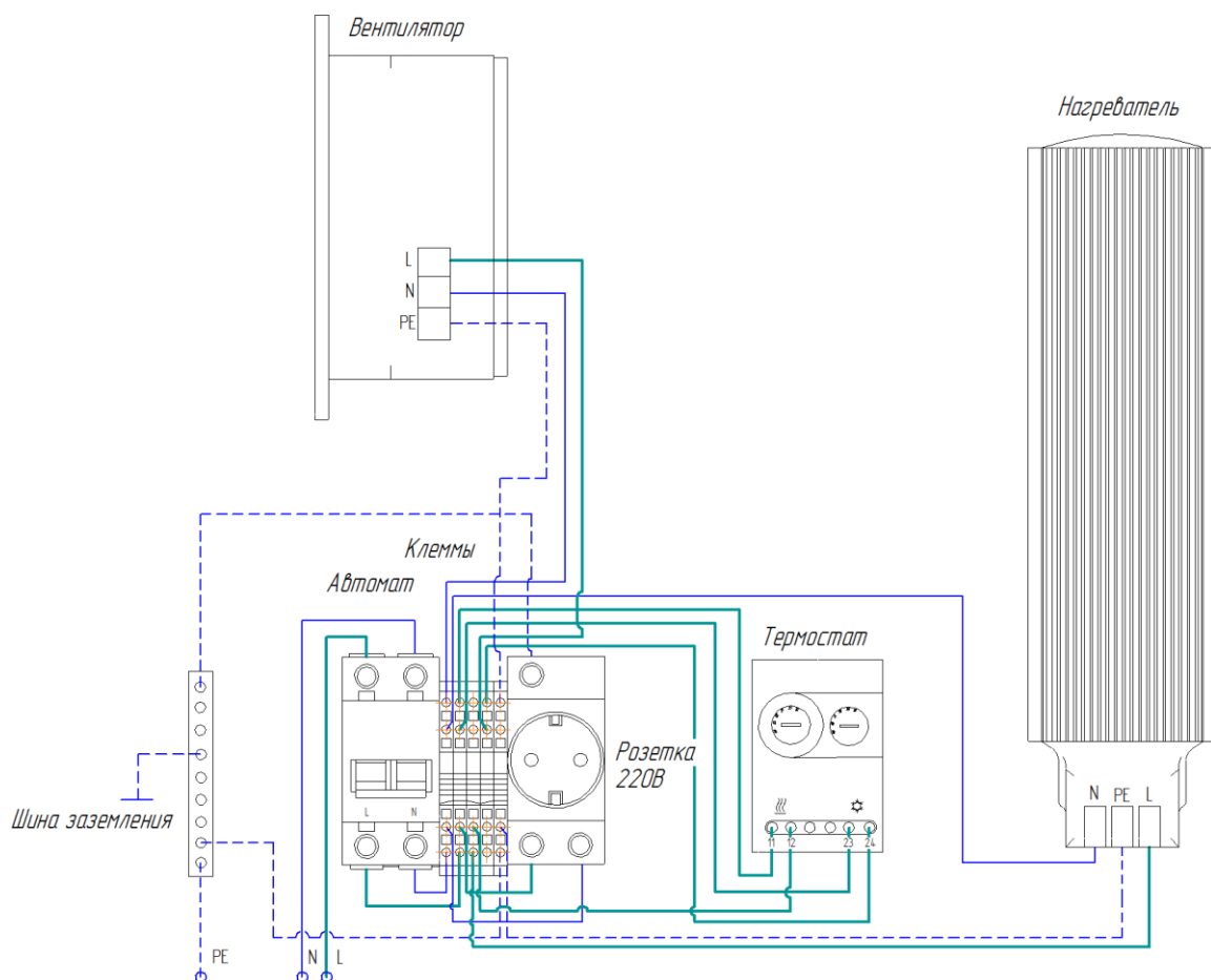
Рисунок 2– Схема подключения SRT05
