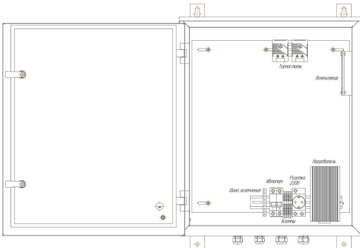
Рисунок 2 – Внешний вид SRT05 (дверь открыта).
